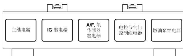
继电器支架 (左驾车型)
