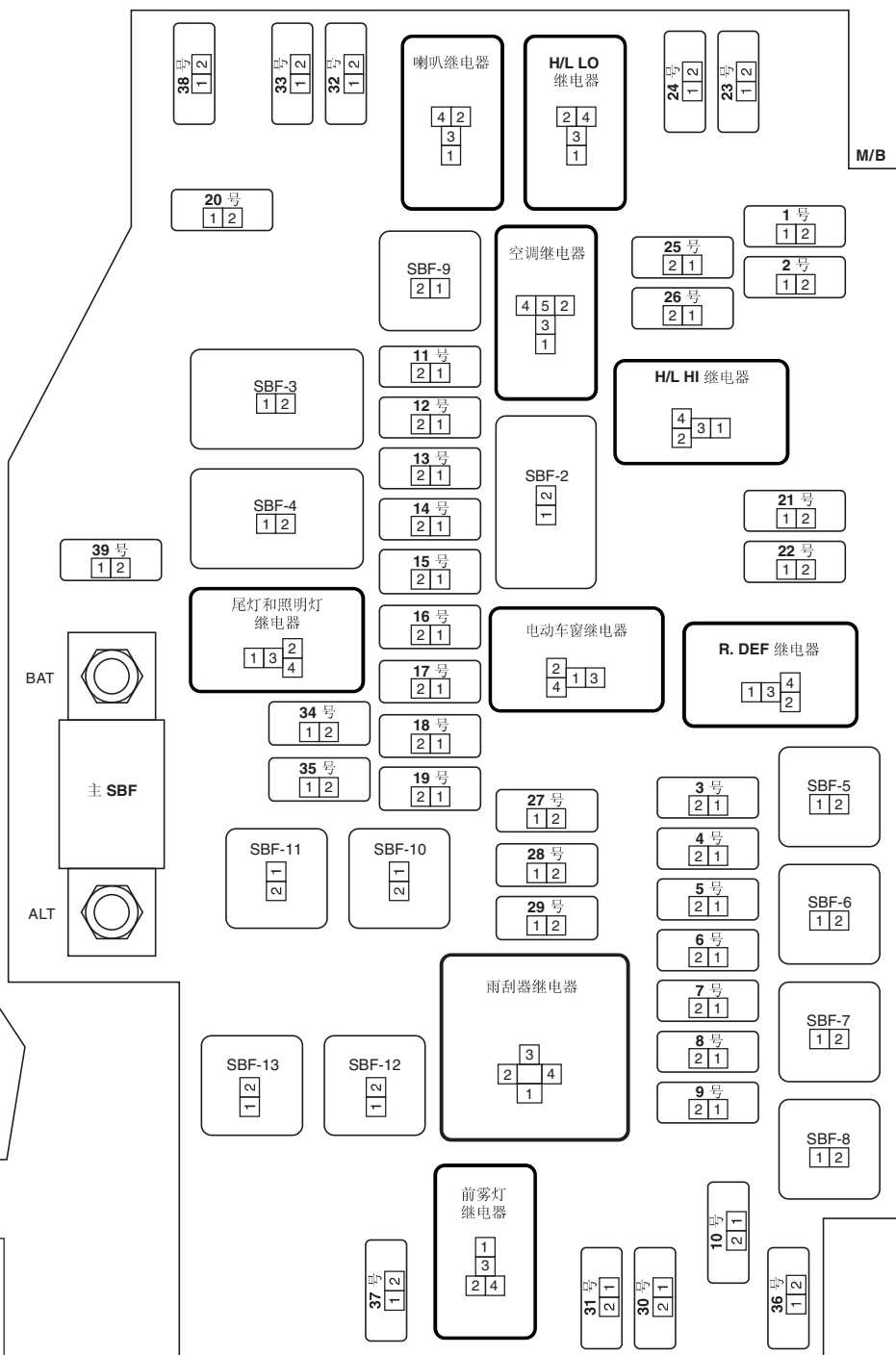
空调继电器支架 (2.0 L 车型)
