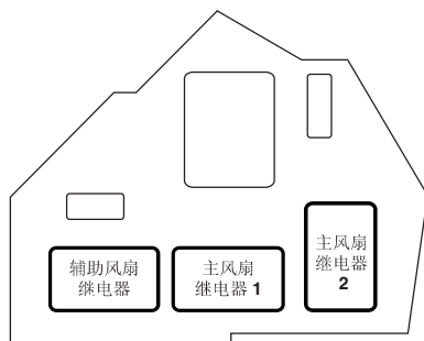
空调继电器支架 (2.5 L 车型)
