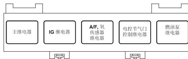
继电器支架 (右驾车型)
